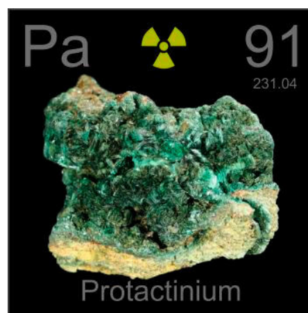
Figura 6. Protactinio.
